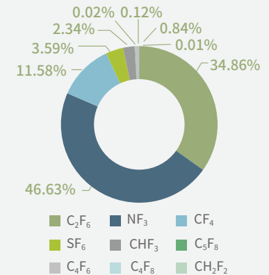
2019 年 PFC 排放二氧化碳當量狀況
