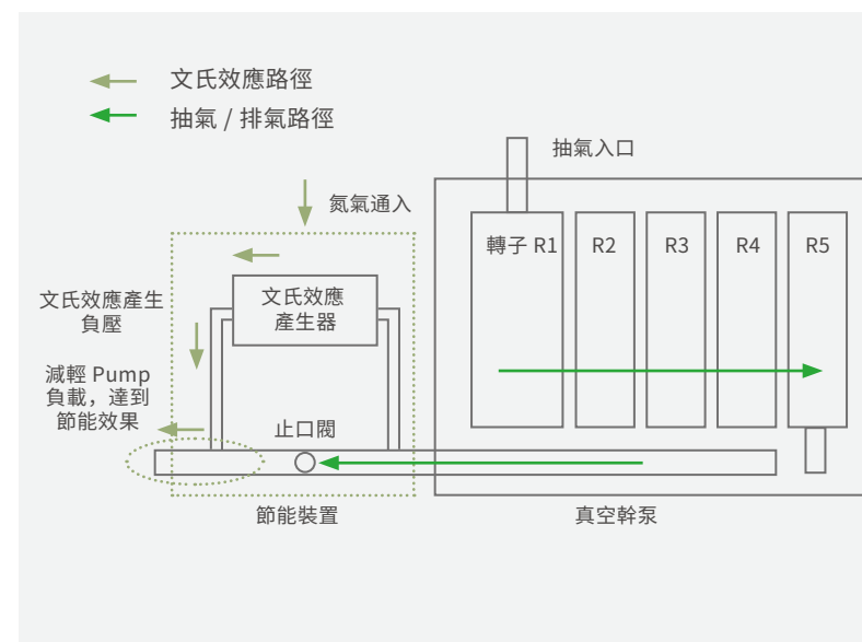
真空泵節能原理示意圖
